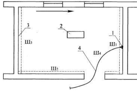
Рис. 22. Схема организации рабочего места звена № 1
