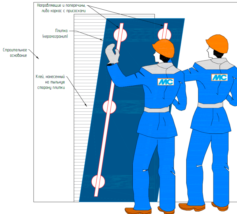
Рис. 31. Монтаж крупноформатного керамогранита
