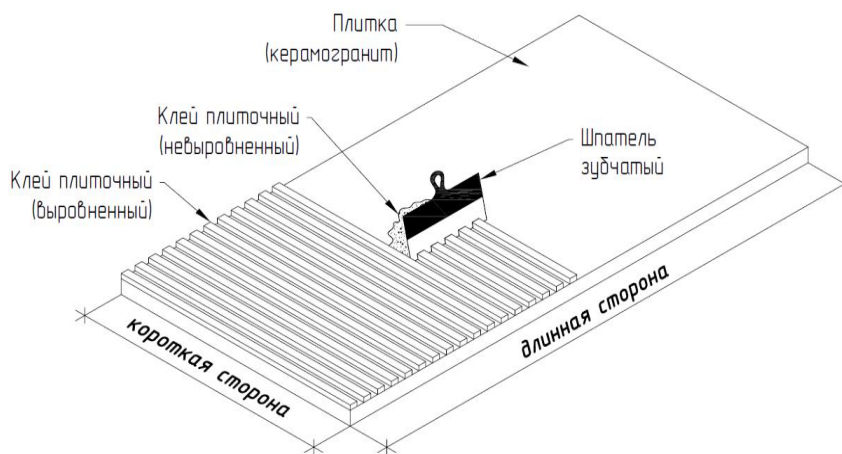
Рис. 26. Нанесение плиточного клея на плитку
