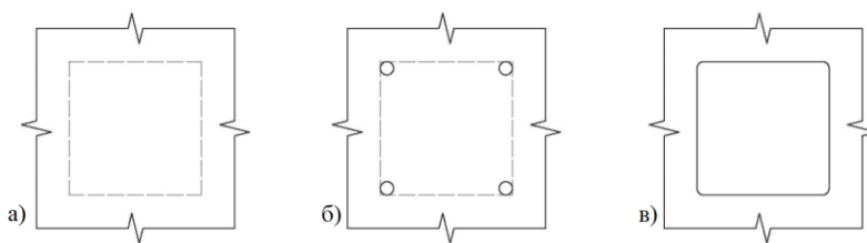
Рис. 30. Резка прямоугольных отверстий
