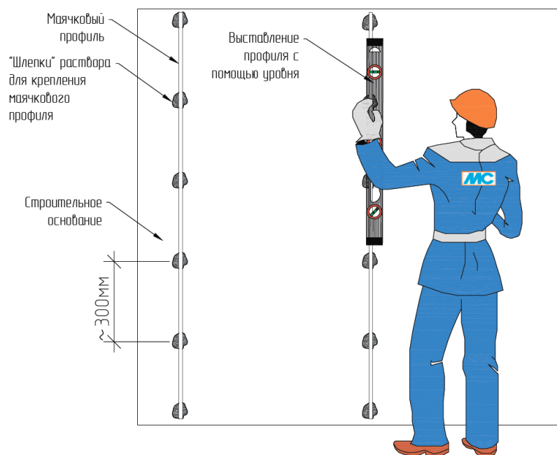
Рис.18. Монтаж маяка с помощью правила с уровнем
